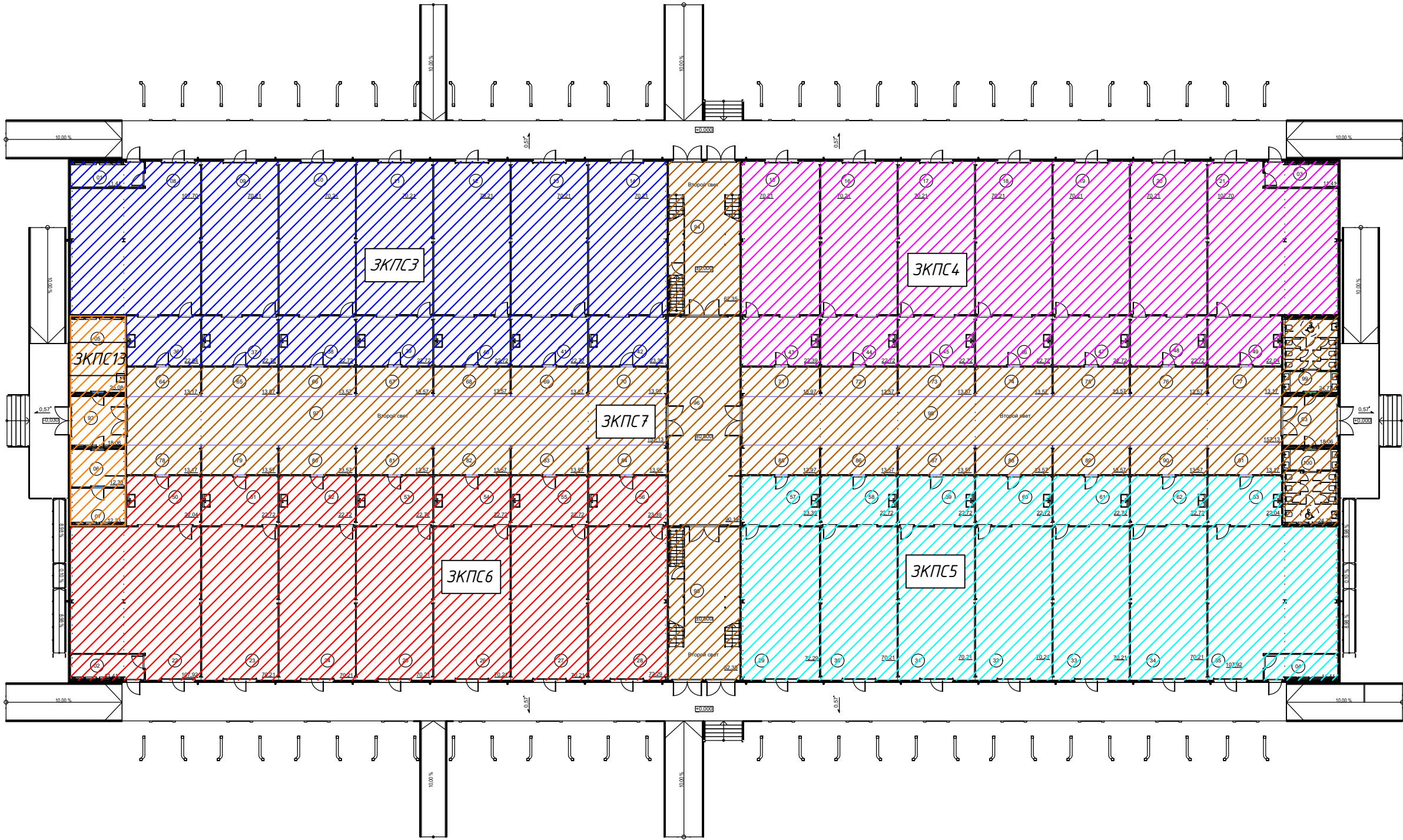
План расположения зон ЗКПС на 1-м этаже
