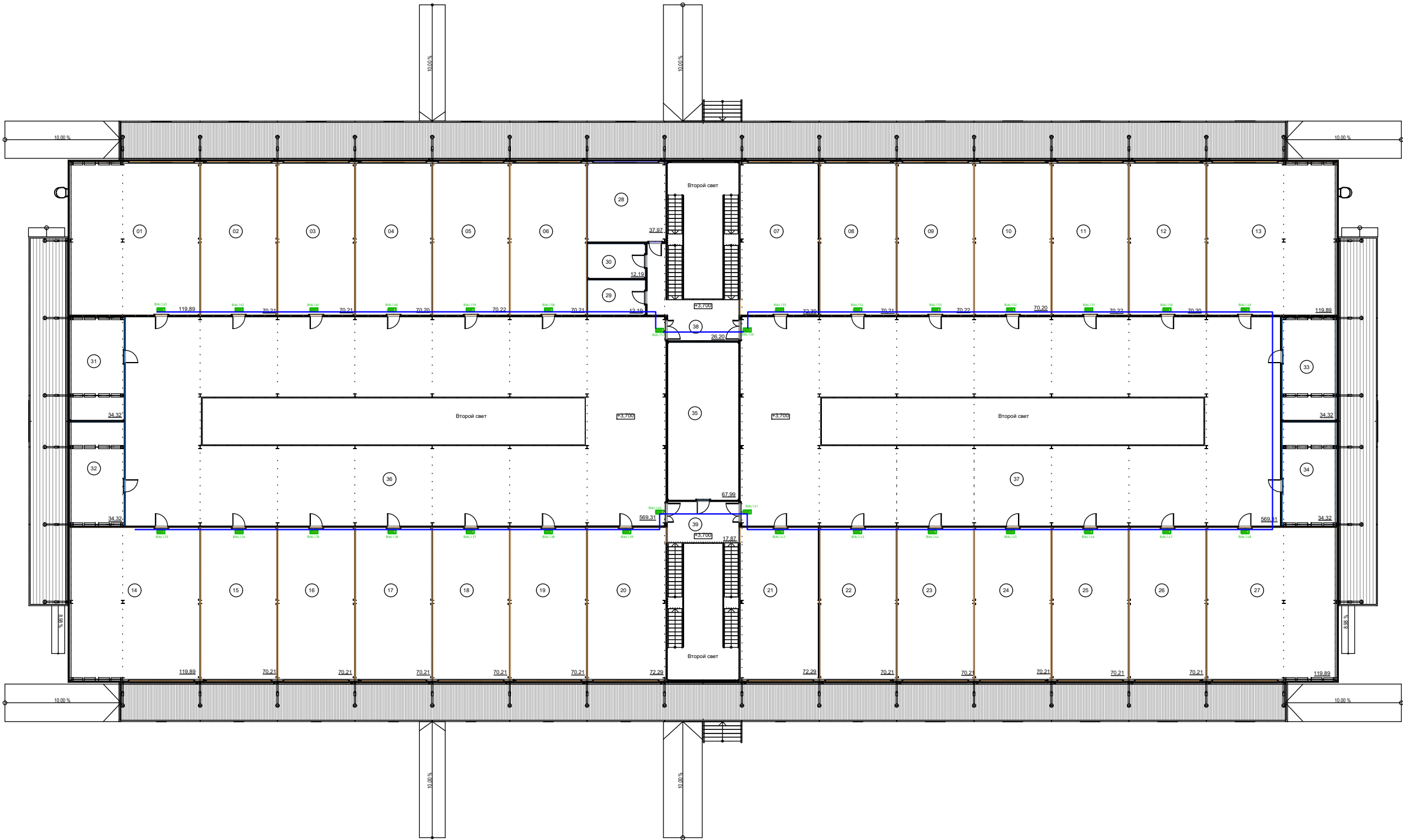
План расположения оборудования и кабельных трасс системы светового оповещения 2-м этаже
